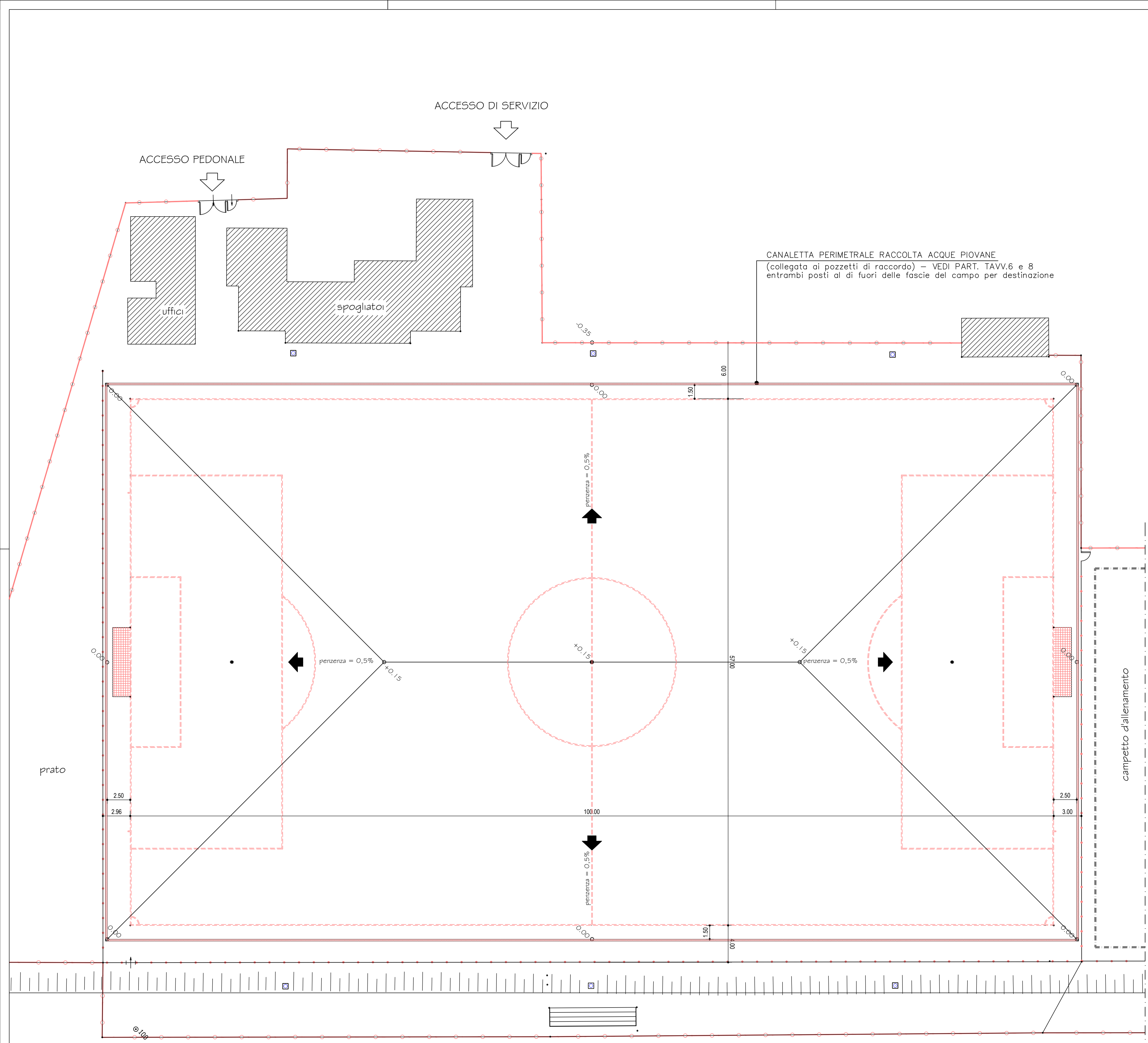
PLANIMETRIA CAMPO DA CALCIO - scala 1:200
