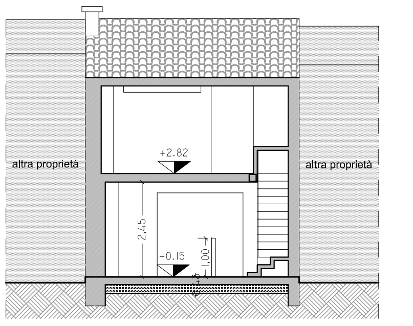
SEZIONE C-C
