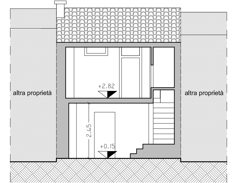
SEZIONE C-C
