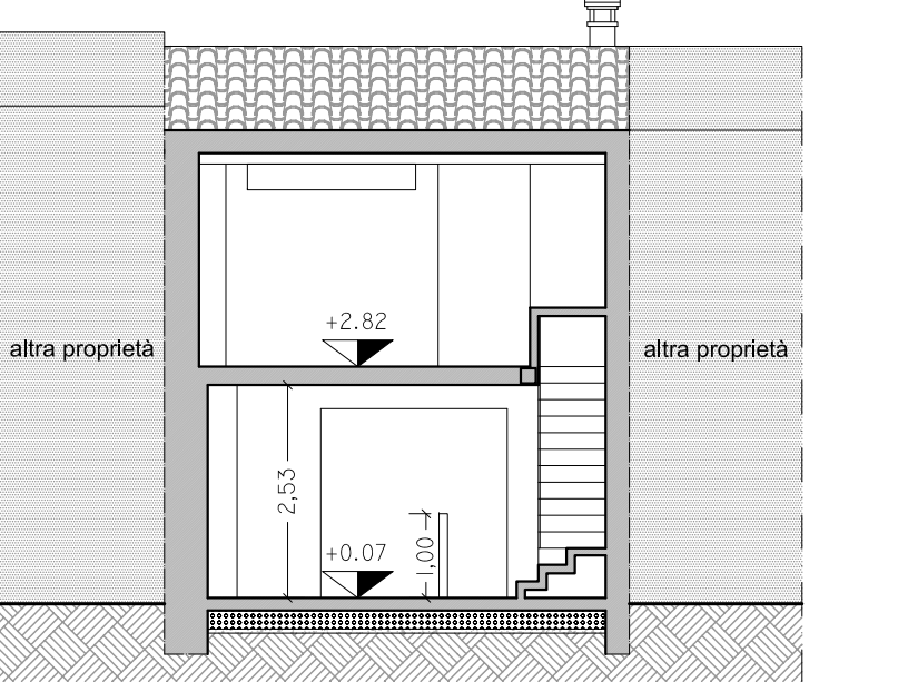
SEZIONE C-C
