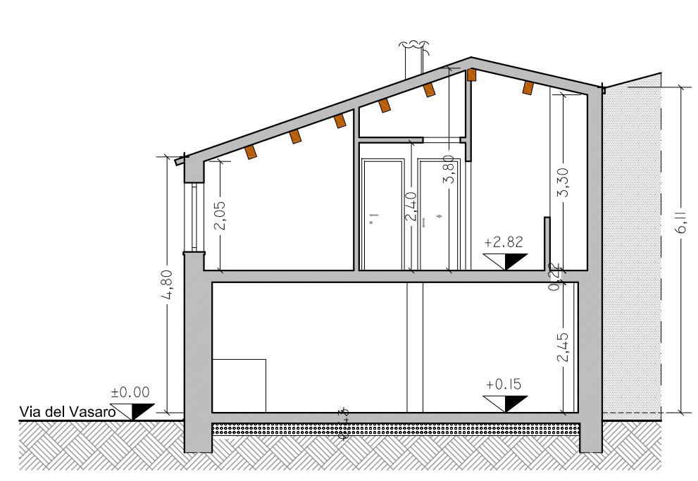
SEZIONE B-B
